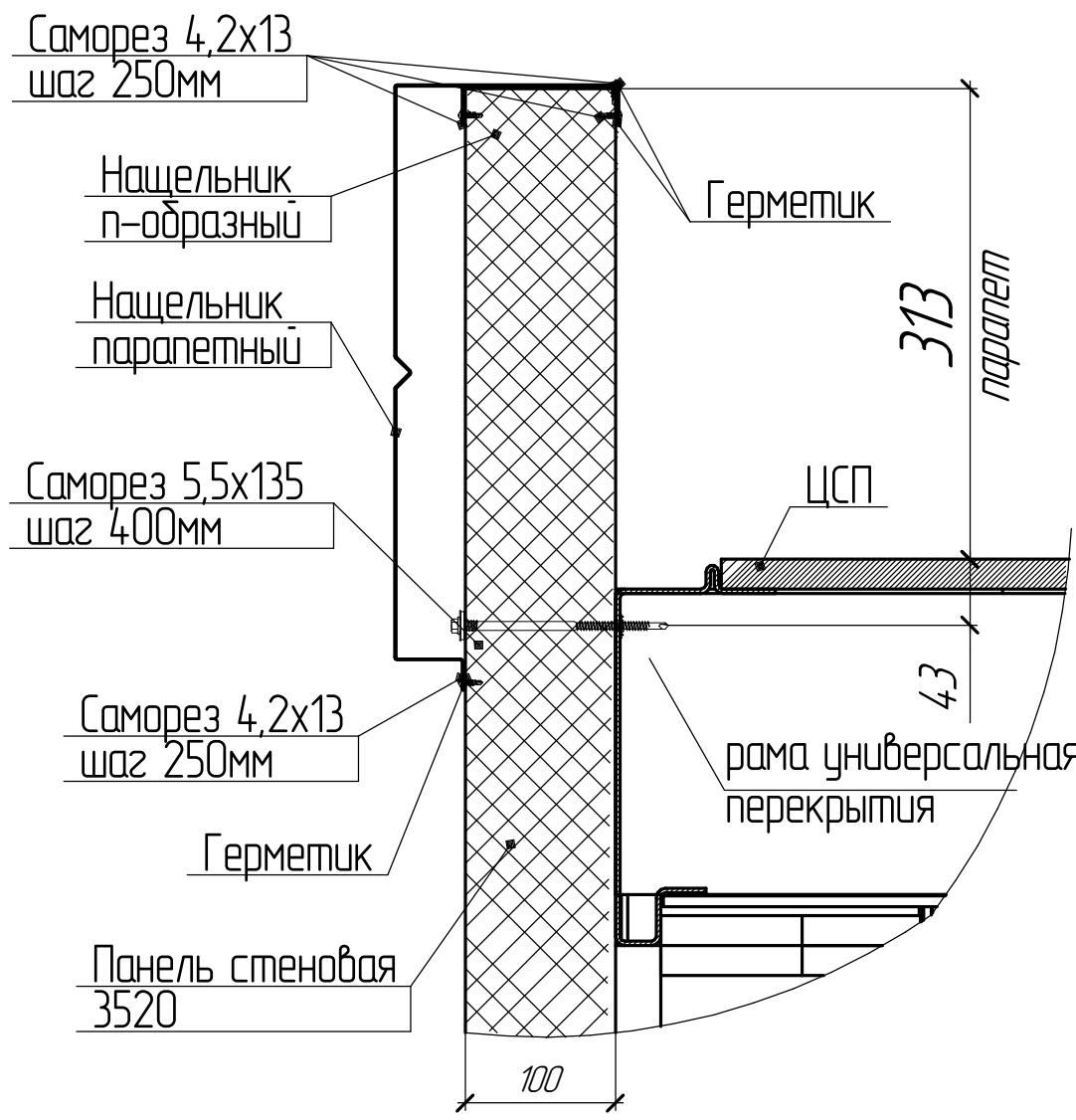
Узел А Узел парапета
