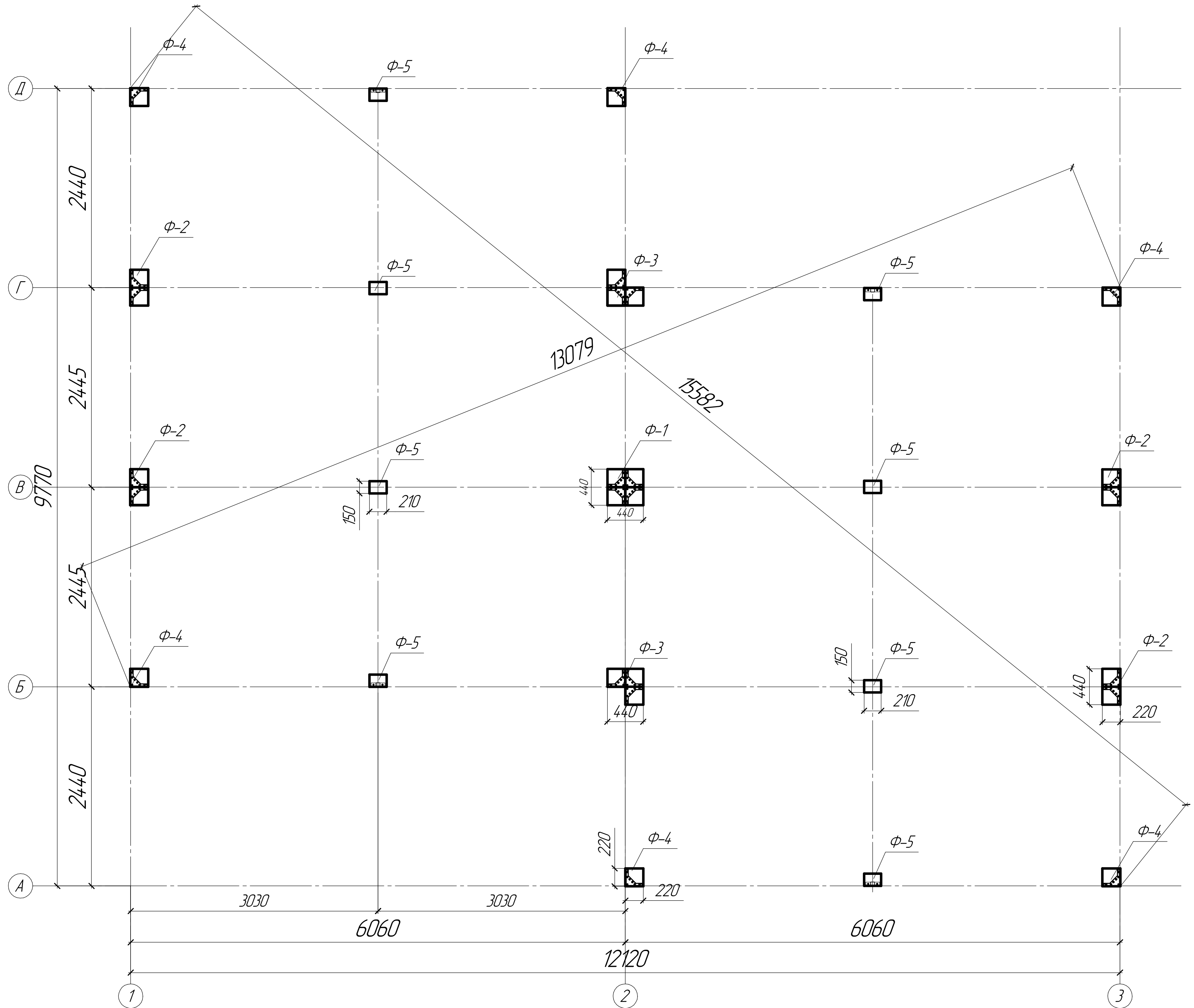
План опорных пластин (М 1:40)
